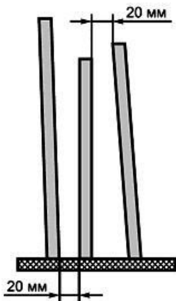
Рисунок 3 - Рекомендуемое расстояние между стеклами
