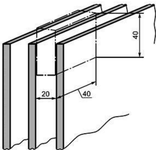
Рисунок 2 - Пример вертикальной установки стекла
