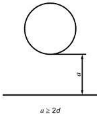
Рисунок 13 - Расстояние от кромки стекла до кромки отверстия
