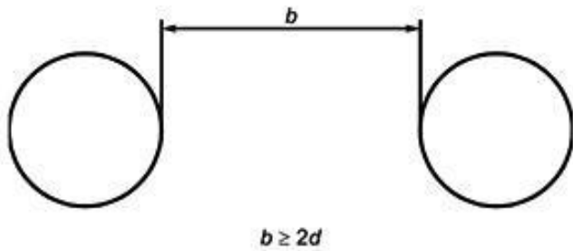
Рисунок 14 - Расстояние между кромками двух отверстий
