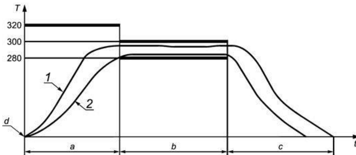
Рисунок 1 - Цикл термической выдержки
