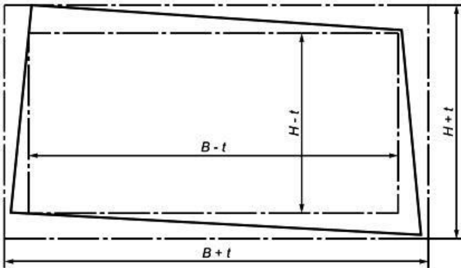
Рисунок 5 - Предельные отклонения по размерам листов стекла
